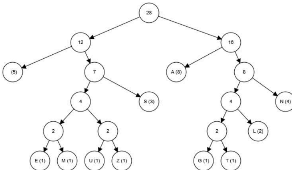
Árbol de Huffman:
